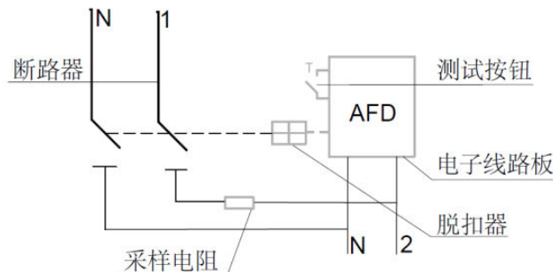
图 1 工作原理图
