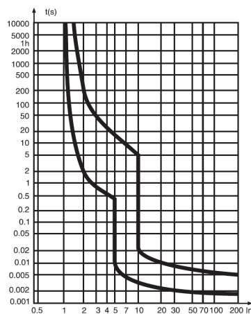
图 3 C 型热/电磁脱扣特性曲线
