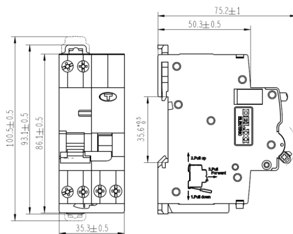
图 4 外形及安装尺寸
